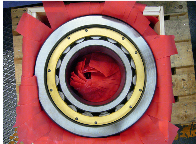
Kırmızı plastik folyo kesilirken dış bilezikte kesik parçalar oluşmuş. Dış bilezik çok yumuşak ve iç bilezik çok sert, kafes yapısı uygunsuz – arıza çıkarmak üzere üretilmiştir.
